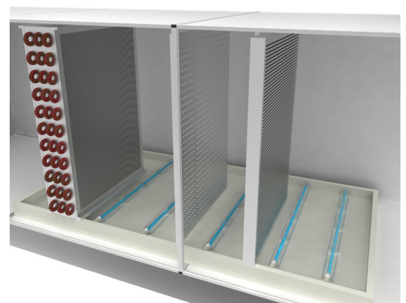
A.H.U. Application
